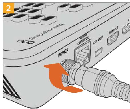
ATEM Mini와 연결되는 커넥터 나사링을 단단히 고정하세요.
